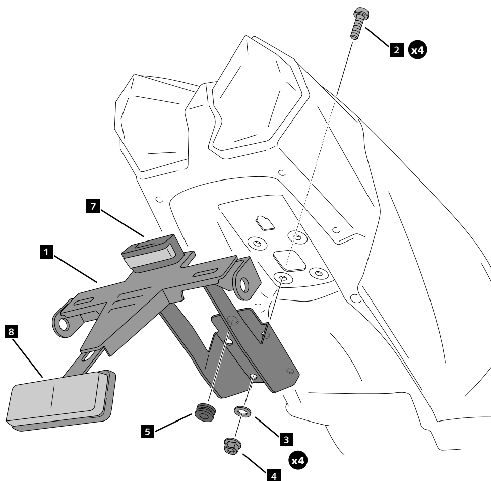
Fijación giro portamatriculas (2 OPCIONES A-B) Fixation license support rotation (2 OPTIONS A-B)
