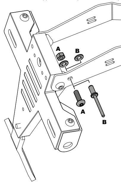
Fijación giro portamatriculas (2 OPCIONES A-B) Fixation license support rotation (2 OPTIONS A-B)
